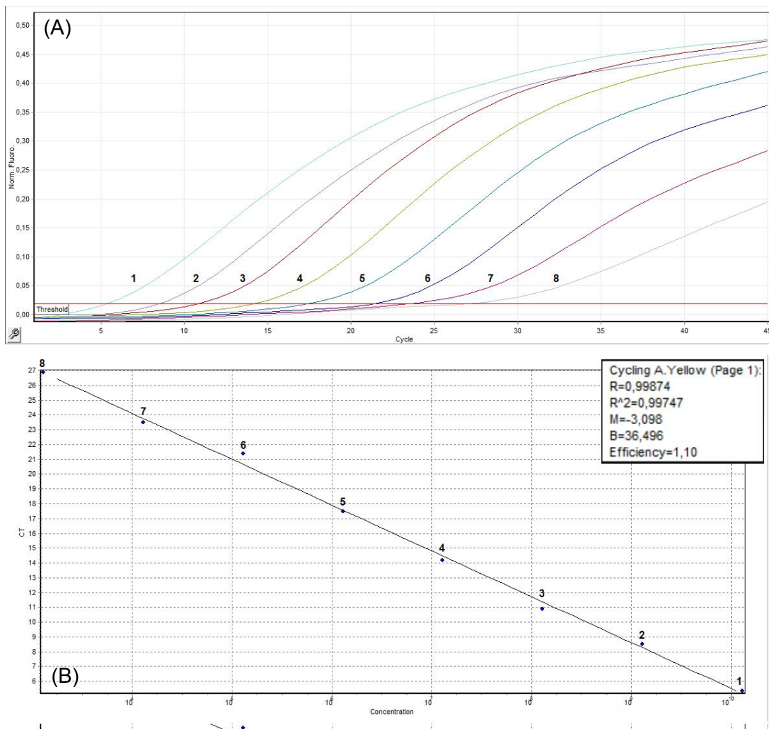
Figura 34: Padronização da curva-padrão para o gene rrs de Bacteroidales suínos (A) Perfil de amplificação da curva padrão com iniciador específico; (B) Curva padrão para quantificação do marcador de Bacteroidales suínos. (1) Diluição 10^0 ; (2) Diluição 10^{-1} ; (3) Diluição 10^{-2} ; (4) Diluição 10^{-3} ; (5) Diluição 10^{-4} ; (6) Diluição 10^{-5} ; (7) Diluição 10^{-6} ; (8) Diluição 10^{-7} .
