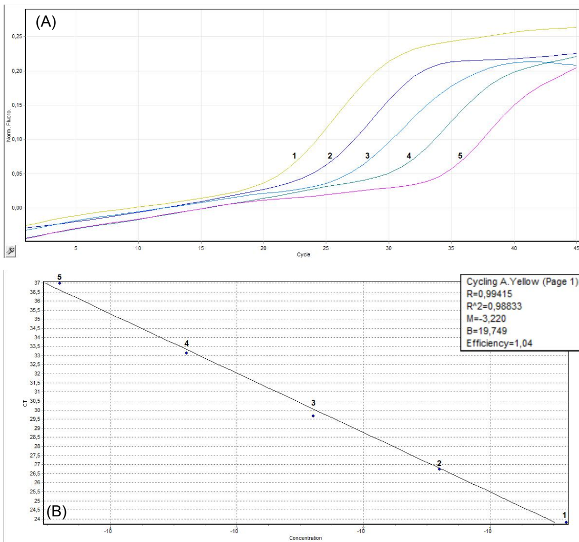
Figura 30: Padronização da curva-padrão para o IPC (A) Perfil de amplificação da curva padrão do IPC. (B) Curva padrão do IPC. (1) Diluição 10^0 ; (2) Diluição 10^{-1} ; (3) Diluição 10^{-2} ; (4) Diluição 10^{-3} ; (5) Diluição 10^{-4} .
