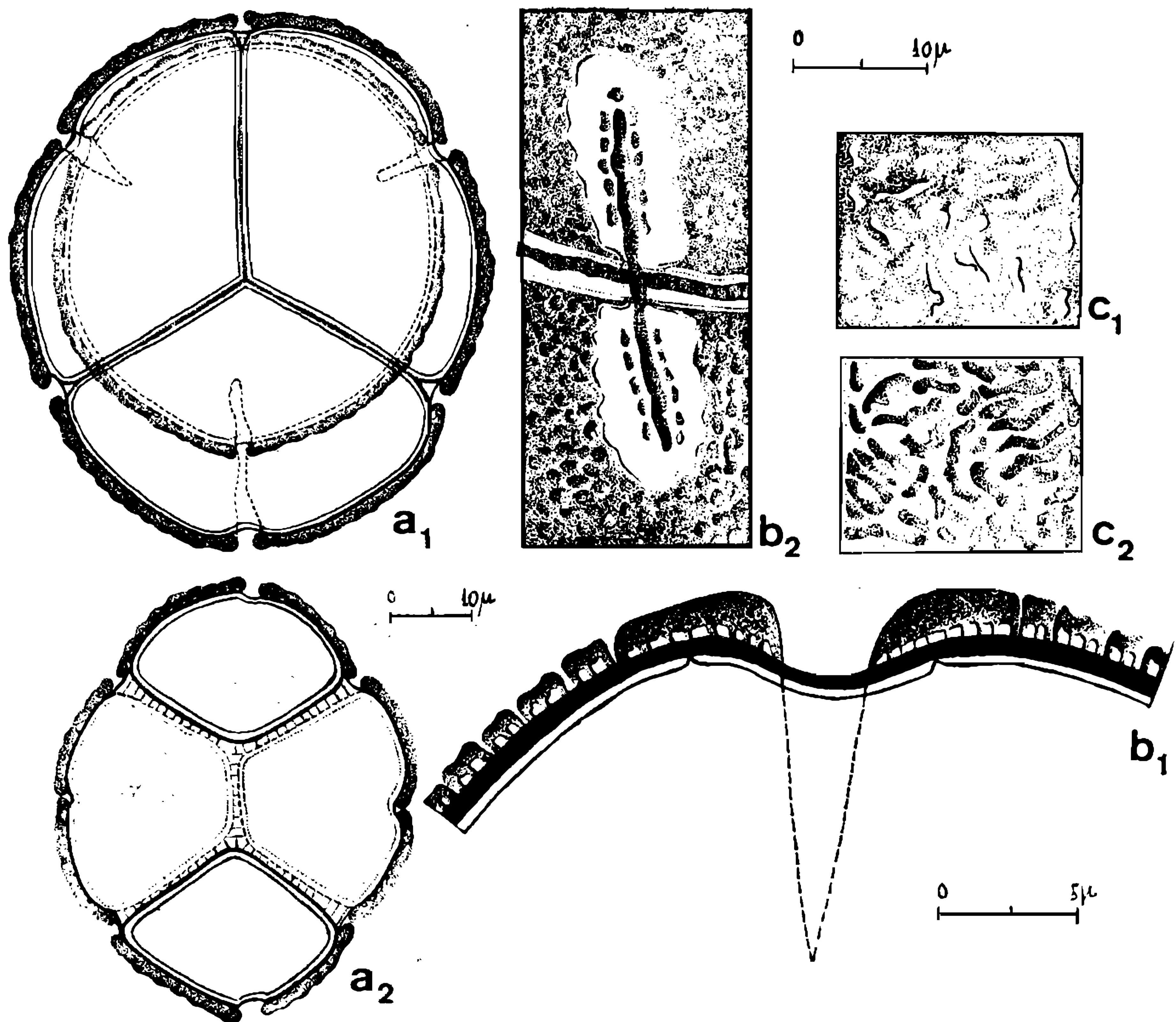
Fig. 4 — Gaylussacia brasiliensis . a 1 = tétada tetraédrica em vista polar, corte óptico; a 2 = tétada tetraedral em vista polar, corte óptico; b 1 = corte transversal pela exina e pelo centro de um colpo (não há espessamento da nexina 1); b 2 = aspecto da superfície da região de um colpo, notando-se no centro da figura a união de dois grãos adjacentes através do concrecimento de seus báculos; c 1 e c 2 = aspecto da superfície em L.O. alto e baixo respectivamente.
