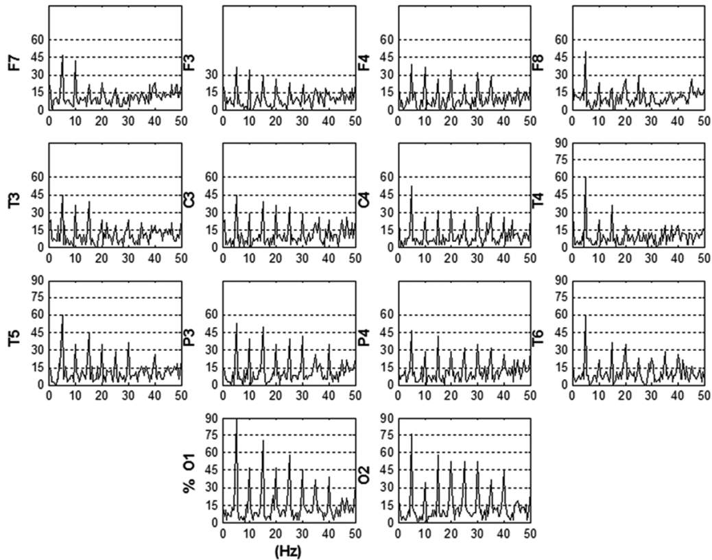
Figura 6. Percentual de detecção de resposta ( TFE(f) \geq TFE_{crit} ) em função da frequência, para as 14 derivações EEG e para os 38 voluntários estimulados com FEI de 5 Hz. Figure 6. Group percentage (38 subjects) of response detection (SFT ( f) \geq SFT_{crit} ) as a function of frequency, for the 14 EEG derivations during IPS of 5 Hz.
