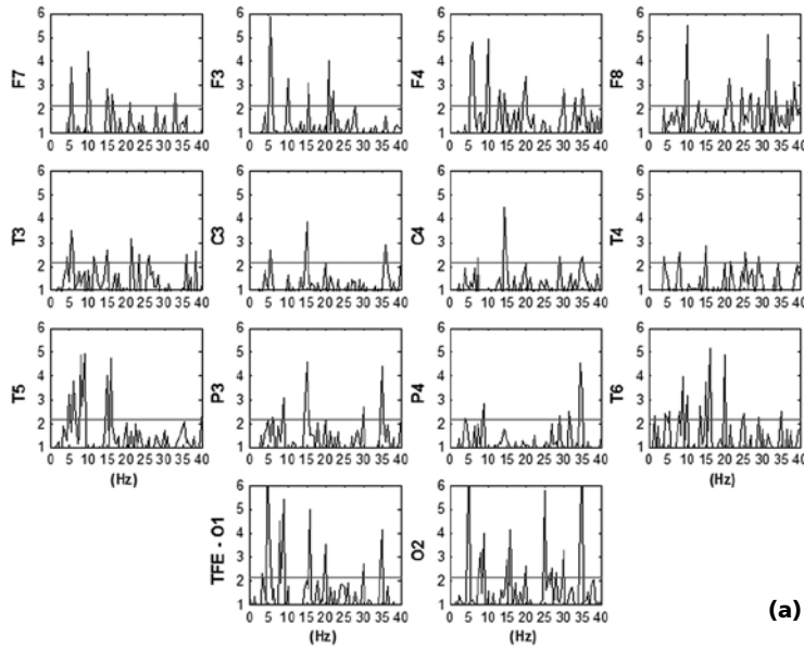
Figura 5. TFE ( f ) do voluntário #31 nas 14 derivações EEG; frequência de FEI de: (a) 5 Hz, (b) 8 Hz e (c) 12 Hz. Em cada gráfico tem-se o valor TFE (ordenada, adimensional) versus a frequência (abscissa em Hz), sendo que a linha horizontal indica o valor crítico de 2,12 para o nível de significância \alpha = 5\% . Figure 5. SFT ( f ) for the 14 EEG derivations from subject #31. IPS frequency: (a) 5 Hz, (b) 8 Hz and (c) 12 Hz. For each plot, abscissa: frequency (Hz), ordinate: SFT, horizontal line: critical value 2.12 for a level of significance \alpha = 5\% .
