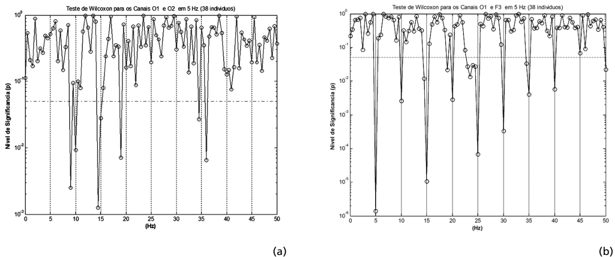
Figura 7. Teste de Wilcoxon (0) do TFE ( f ) nas frequências de estimulação de 5 Hz e harmônicos. Valores do teste menores que o nível de significância p = 0.05 (linha horizontal tracejada) implicam na rejeição da hipótese nula de igualdade das medianas. Comparação entre derivações: (a) O1 x O2 e (b) O1 x F3. Figure 7. The Wilcoxon's Test (0) for SFT ( f ) at IPS 5 Hz and harmonics. SFT values lower than the significance level p = 0.05 (horizontal dot-dashed line) imply to reject the null hypothesis of median equality. Comparison between derivations: (a) O1 x O2 and (b) O1 x F3.
