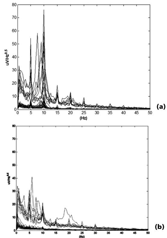
Figura 3. Estimativas espectrais superpostas dos 38 voluntários estimulados a 5 Hz, para derivações (a) O2 e (b) F3. Figure 3. Superposed spectra of 38 subjects stimulated at 5 Hz, derivations (a) O2 and (b) F3.
