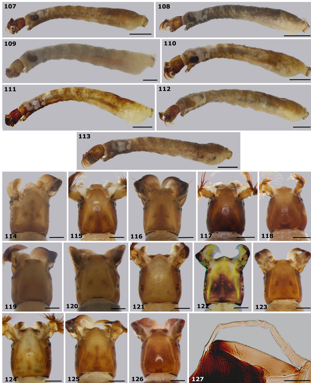
Figs 107–127. 107–113. Larvas (last instar). 107–108. Simulium ( Anasolen ) Enderlein, 1930. 107. dentulosum Roubaud, 1915. 108. imerinae Roubaud, 1905. — 109. S. ( Freemanellum ) manense Elsen & Escaffre, 1976. — 110. S. ( Hearlea ) canadense Hearle, 1932. — 111. S. ( Hemicnetha ) paynei Vargas, 1942. — 112. S. ( Shewellomyia ) pictipes Hagen, 1880. — 113. S. ( Obuchovia ) auricoma Meigen, 1818. — 114–126. Last instar larvae. Head, dorsal view. 114–118. S. ( Anasolen ). 114. ambositrae Grenier & Grjebine, 1959. 115. dentulosum . 116. imerinae . 117. masabae Gibbins, 1934. 118. nili Gibbins, 1934. — 119–120. S. ( Freemanellum ). 119. manense . 120. hirsutilateris De-Meillon, 1937. — 121. S. ( Hearlea ) canadense . — 122–123. S. ( Hemicnetha ). 122. brachycladum Lutz & Pinto, 1932. 123. paynei . — 124–125. S. ( Shewellomyia ). 124. claricentrum Adler, 1990. 125. pictipes . — 126. S. ( Obuchovia ) ibericum Crosskey & Santos Grácio, 1985. — 127. Antenna of S. ( Anasolen ) ambositrae . Scale bars: 107–113 = 1 mm; 114–126 = 0.5 mm; 127 = 0.2 mm.
