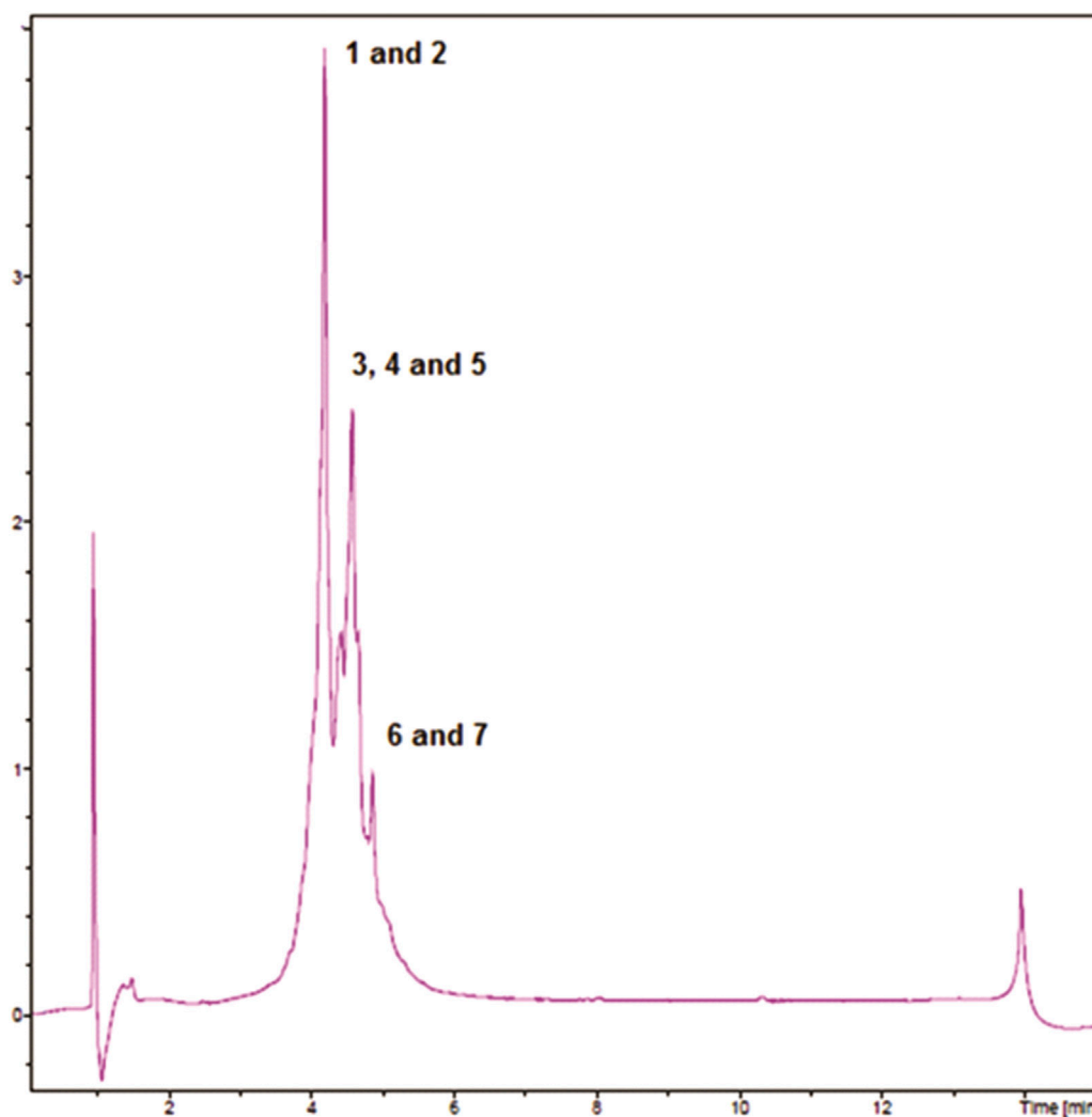
FIGURE 1 RP-UHPLC-DAD profiles of EENL.
