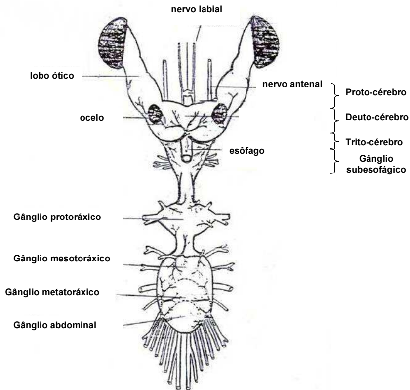
Figura 4: Desenho esquemático do sistema nervoso central de triatomíneos (adaptado de Insausti, 1994).
