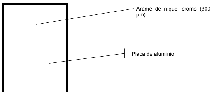
Figura 13: Desenho esquemático da fonte térmica constituída pela placa de alumínio e o arame de níquel-cromo.
