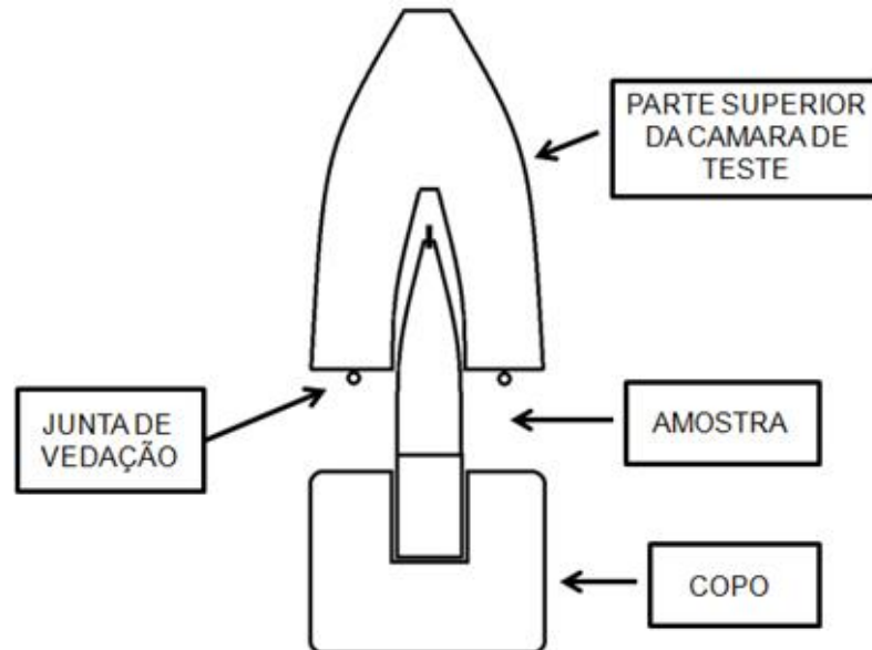
Figura 1.9 – Esquema demonstrativo da câmara de teste
