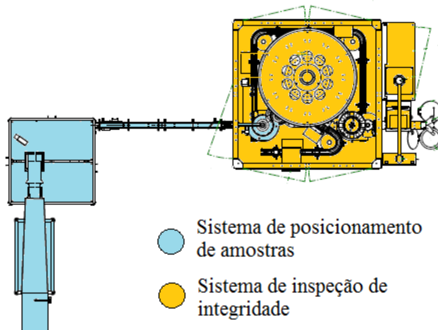
Figura 3.4: Identificação dos sistemas da linha para inspeção de integridade
