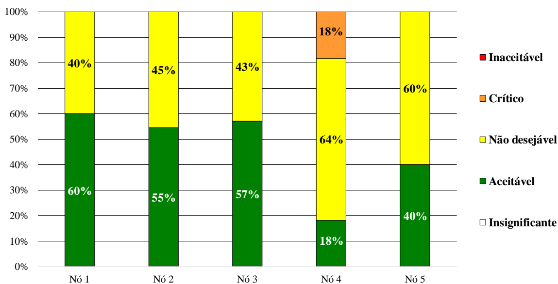
Figura 4.12 – Classificação dos riscos associados aos equipamentos de inspeção de integridade.
