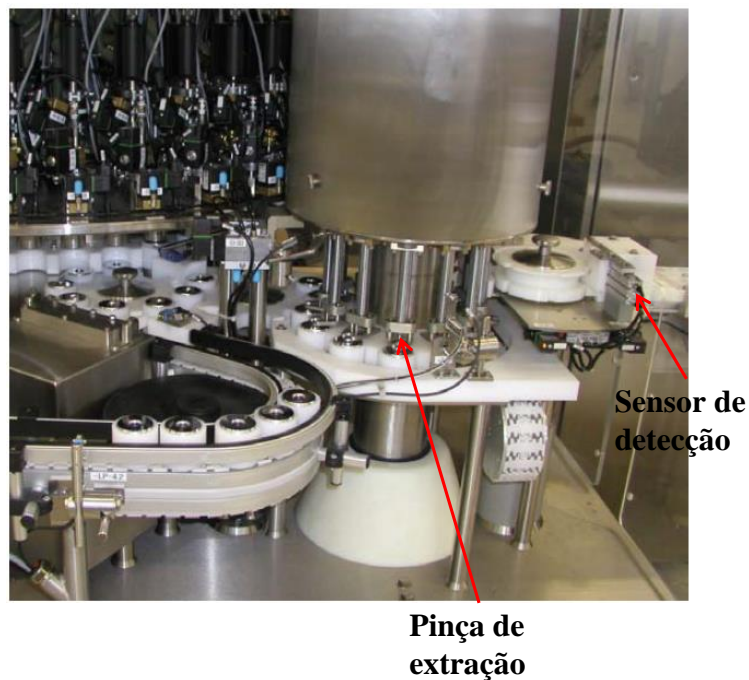
Figura 4.6 – Estação de extração de amostras aprovadas.
