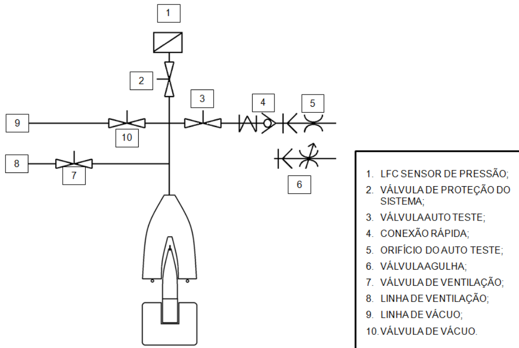
Figura 1.10 – Esquema demonstrativo dos componentes da câmara de teste
