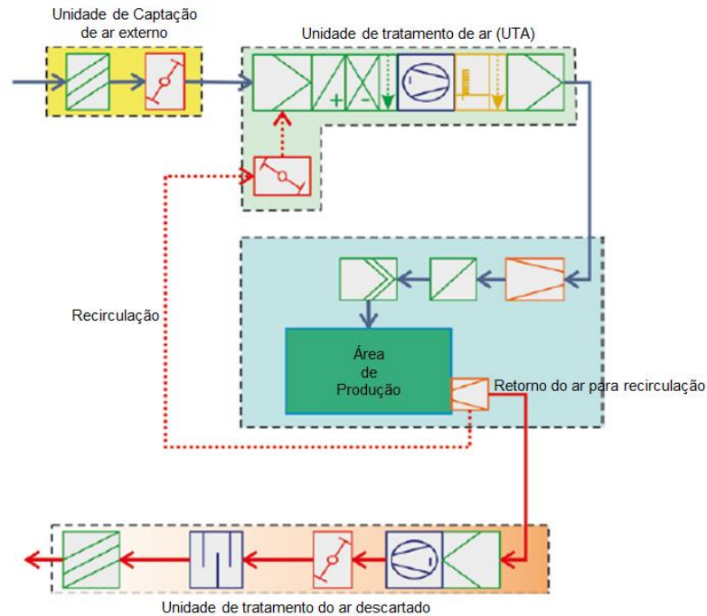
Figura 1.2: Subsistemas que compõem o sistema HVAC (Brasil, 2013).
