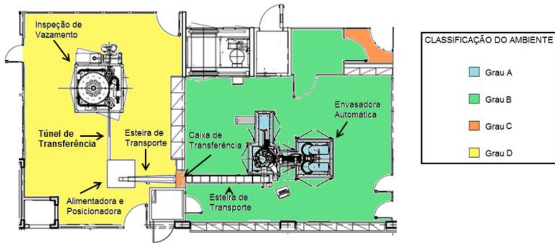
Figura 1.4 - Classificação dos ambientes usados para o envase do imunobiológico e para a realização do teste de estanqueidade (confecção própria).
