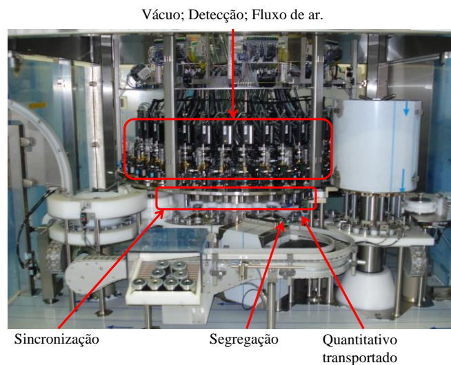
Figura 4.4 - Identificação dos parâmetros de acordo com posicionamento dos componentes da estação central.
