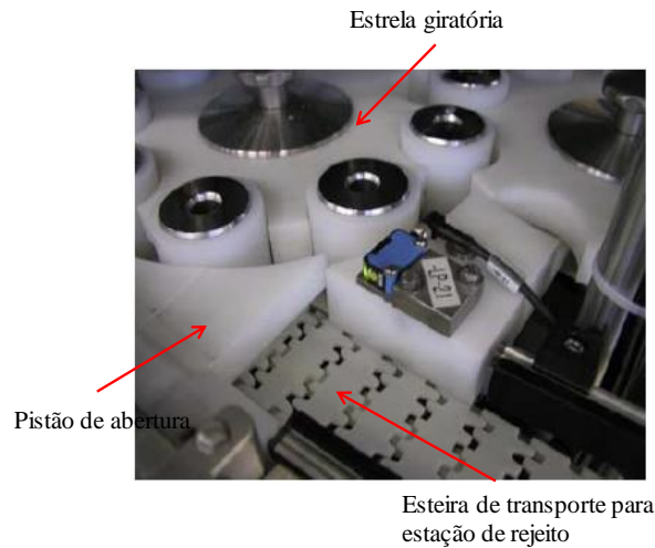
Figura 4.5 – Estrela giratória e estação de rejeito
