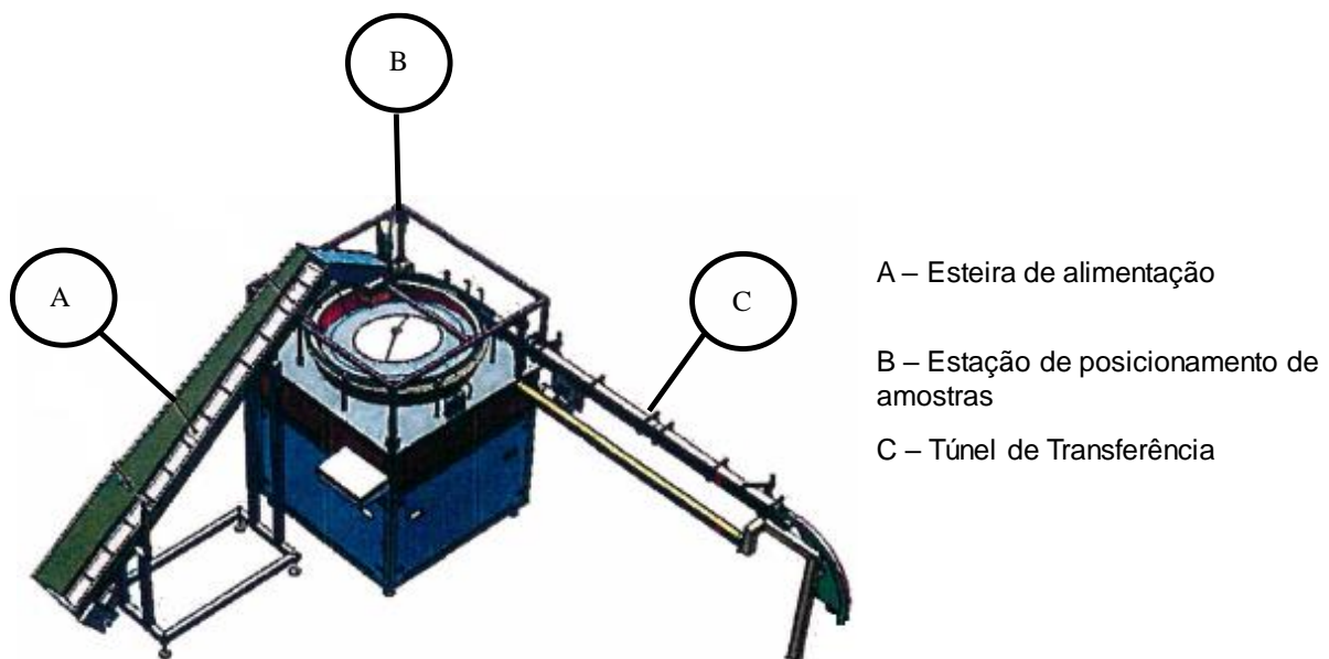
Figura 1.7 – Sistema posicionado de amostras.
