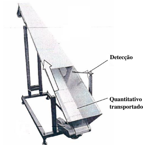
Figura 4.1 – Identificação dos parâmetros de acordo com o posicionamento dos componentes da esteira de alimentação.
