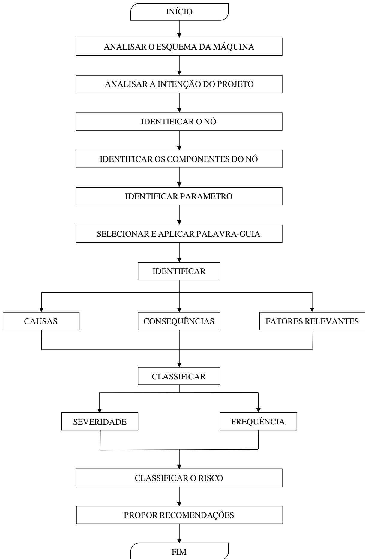
Figura 3.3 – Fluxograma das atividades adotadas para a condução do estudo HAZOP.
