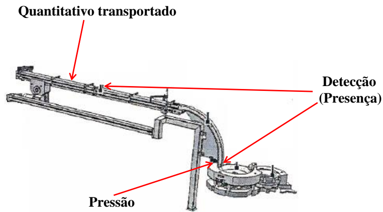
Figura 4.3 – Identificação dos parâmetros de acordo com posicionamento dos componentes do túnel de transferência.
