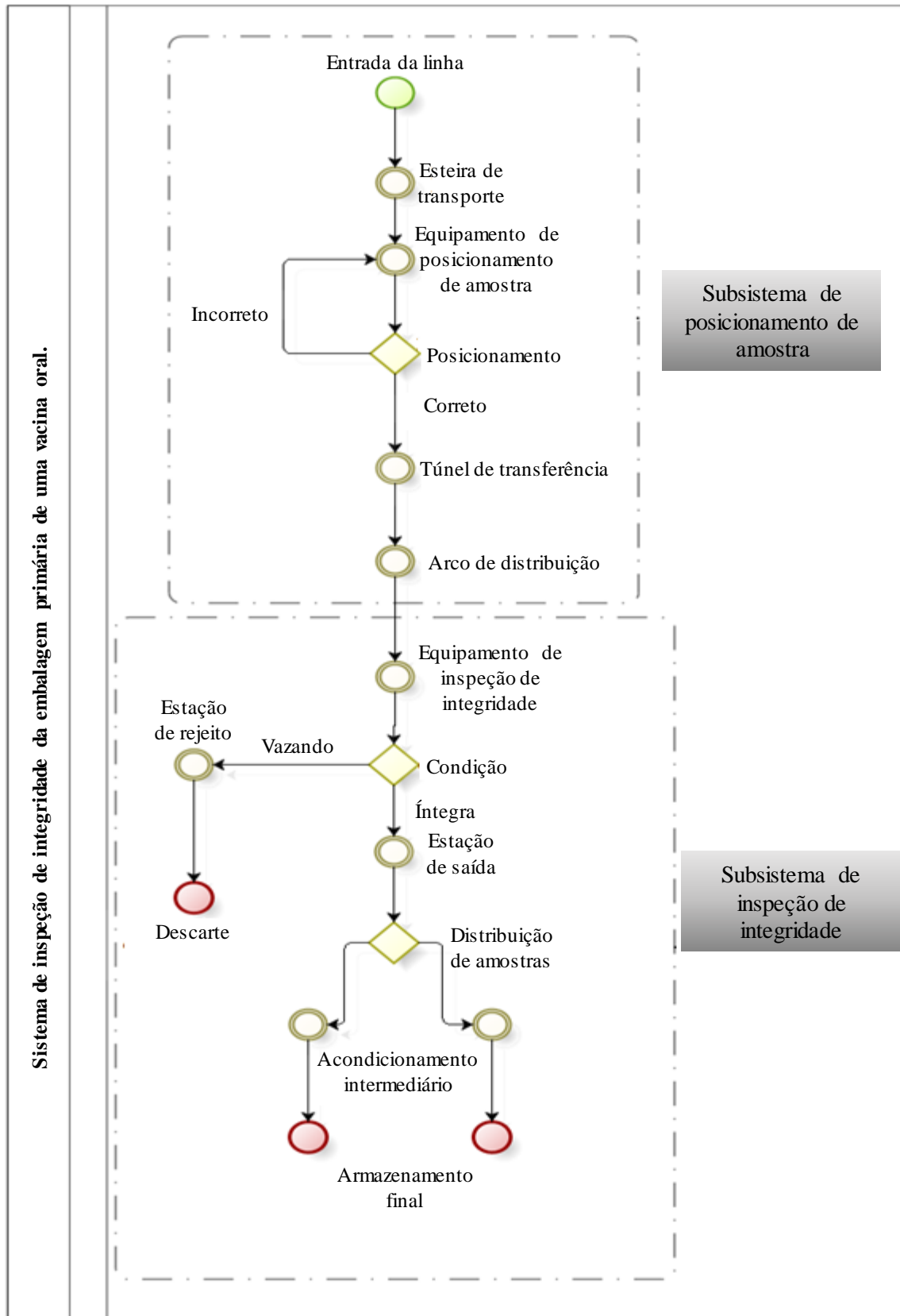
Figura 3.5 – Fluxograma da linha de inspeção de integridade.
