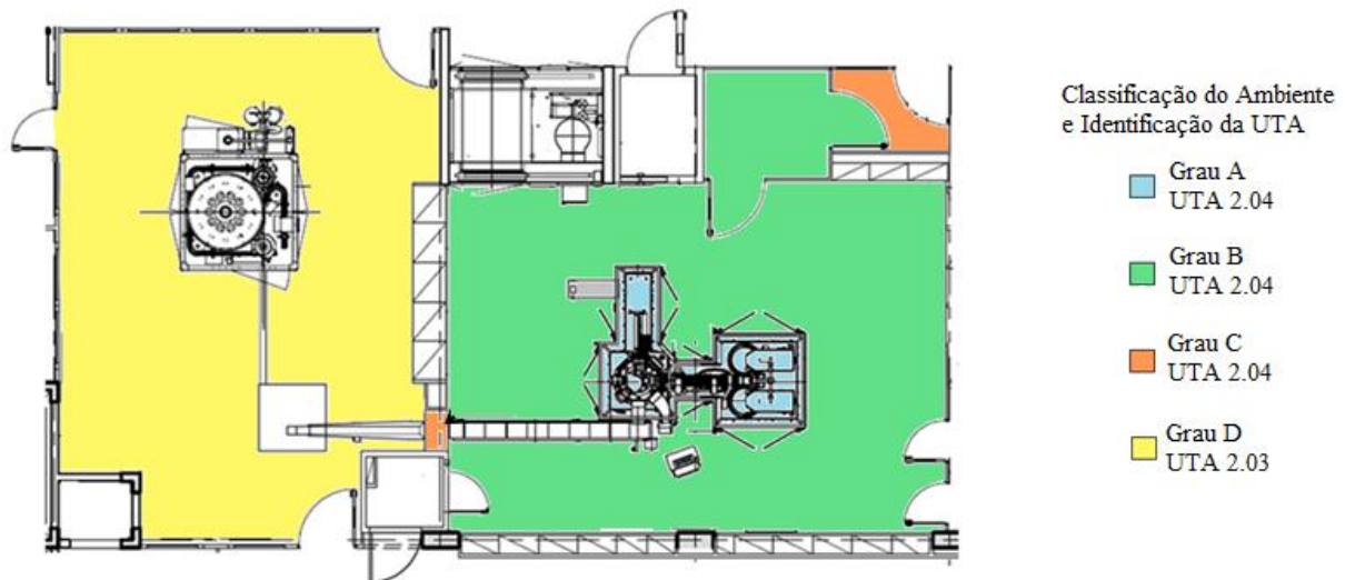
Figura: 3.7 – Classificações do ambiente e identificação da UTA
