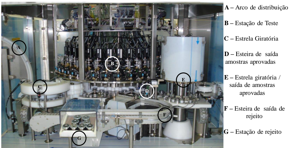
Figura 1.8 – Estação central do equipamento de teste de inspeção.
