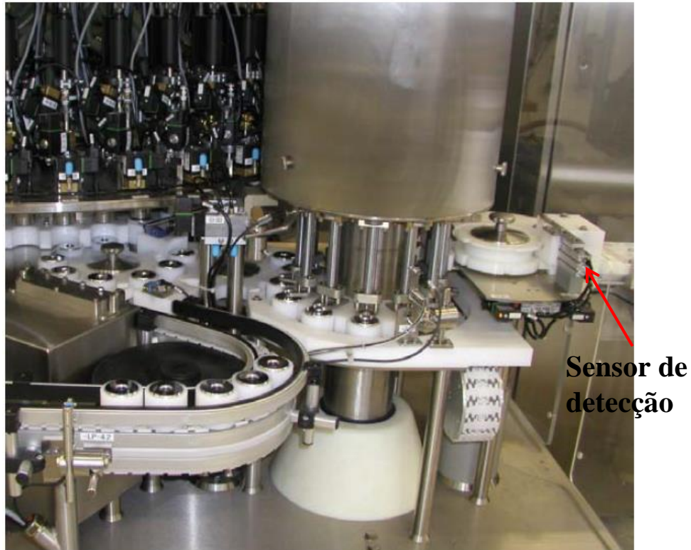
Figura 4.7 – Posicionamento do sensor de detecção de saída de amostra
