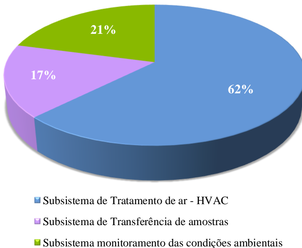
Figura 4.13 – Gráfico representativo da distribuição de percentual dos modos de falhas analisados.
