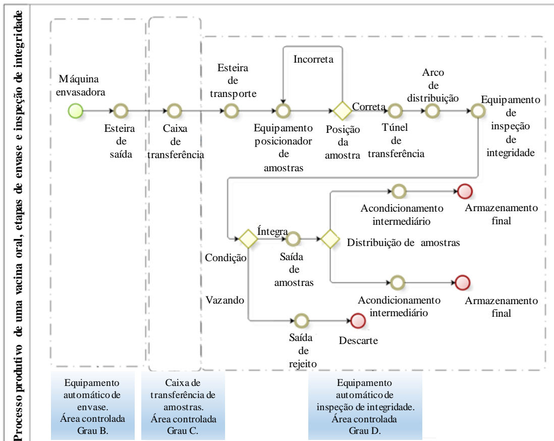
Figura 3.2 – Modelagem do processo envase e inspeção de integridade da primária de uma vacina oral.
