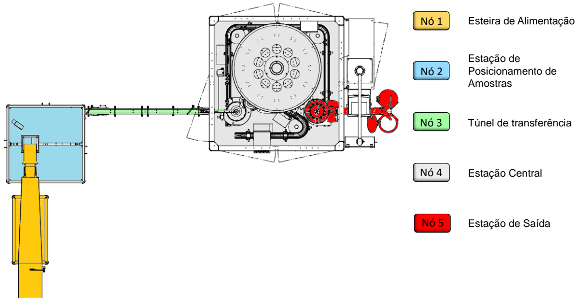
Figura 3.6: Identificação dos nós da linha de inspeção de integridade.
